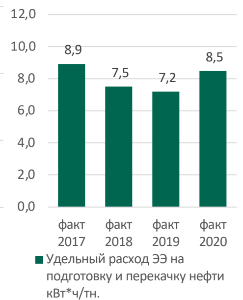
Подготовка нефти
