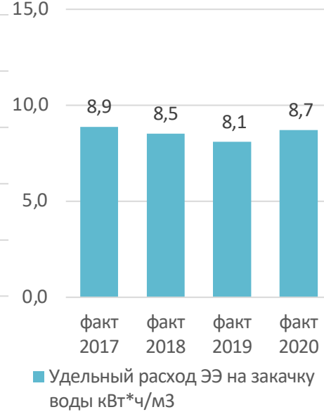
Закачка воды
